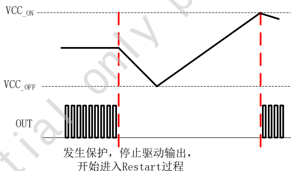
Figure 3. 保护功能工作原理
